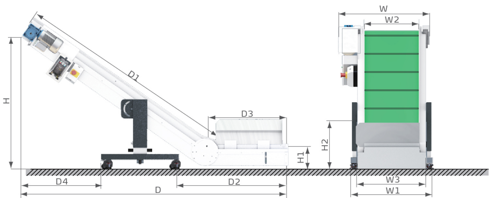
CB系列外形尺寸图
