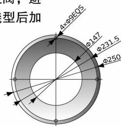
SHR-3U-S 安裝底座
