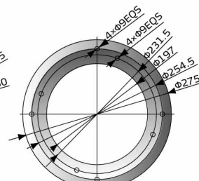
SHR-6U-S~SHR-24U-S 安裝底座
