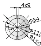
底座安装尺寸
