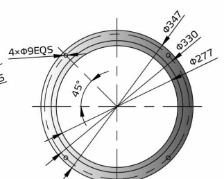
SHR-36U-S~SHR-96U-S 安裝底座
